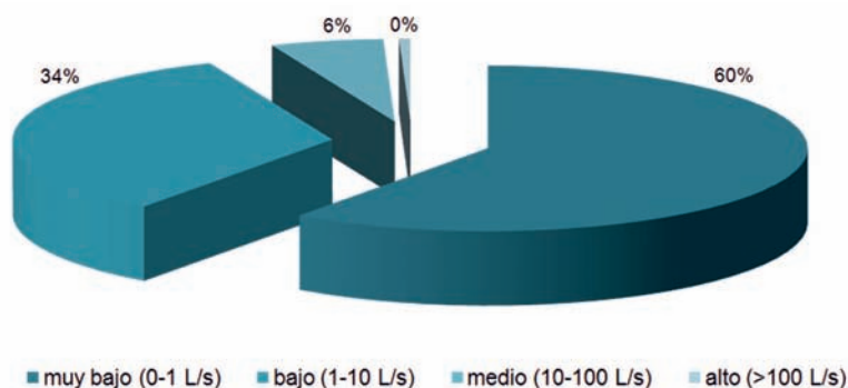
Figura 2. Distribución de caudales de las surgencias catalogadas en CTF hasta el momento para la comarca de las Villas (18 de noviembre de 2013)
