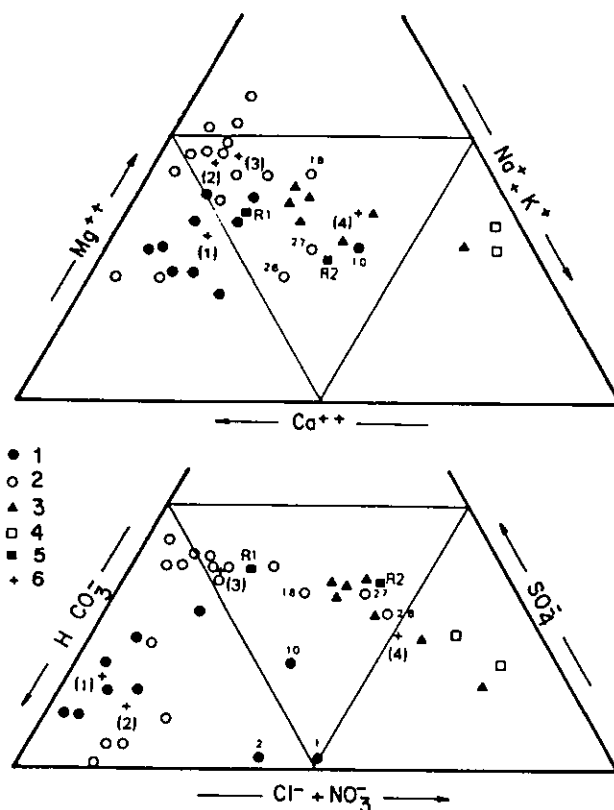
Fig. 2.—Proporciones iónicas de los puntos de agua analizados.— 1: Puntos en relación con metapelitas nevado-filábrides. 2: Puntos en relación con acuíferos alpujárrides. 3: Puntos del acuífero del delta. 4: Muestras de las Albuferas. 5: Muestras de aguas superficiales. 6: Composiciones medias de los grupos de aguas deducidos del análisis «cluster» (más detalles en texto).
