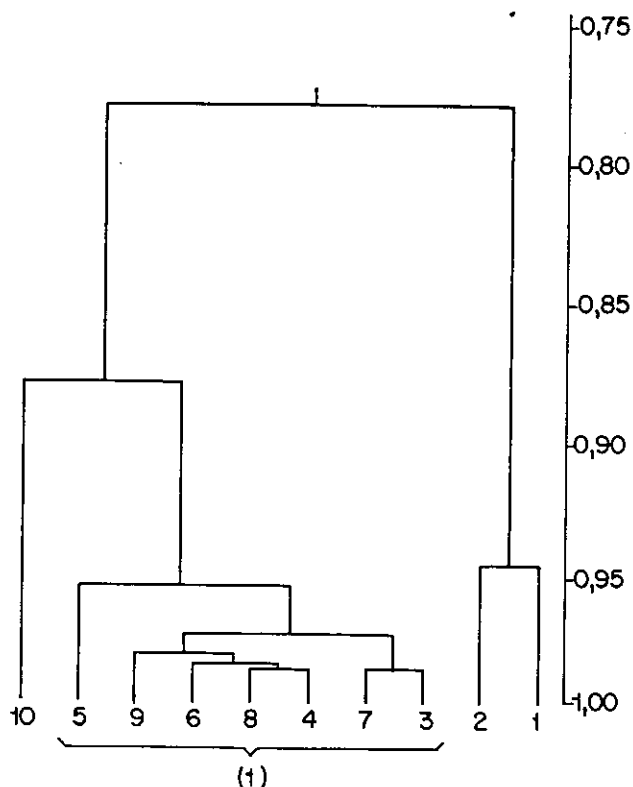
Fig. 4.—Dendrograma correspondiente a los puntos de agua en relación con materiales nevado-filábrides.
