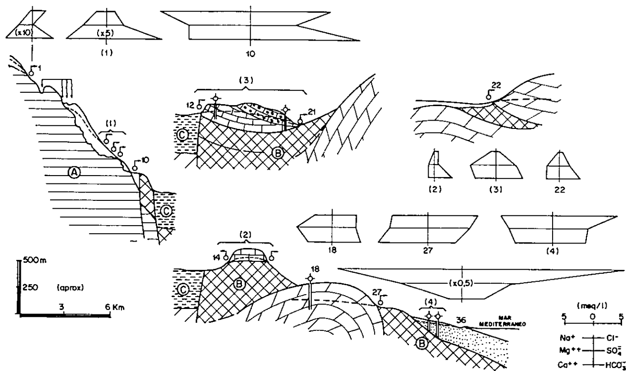
Fig. 3.—Cortes esquemáticos, en dirección aproximada N-S, ilustrativos de la tipología hidrogeológica de los puntos de agua más representativos de la cuenca, acompañados de diagramas hidroquímicos poligonales (algunos de los cuales tienen la escala modificada para facilitar de la representación). Con paréntesis se indican los grupos de puntos afines resultantes del análisis «cluster» (ver texto y leyenda de la figura 1 para más detalles).
