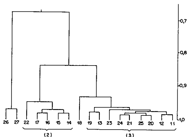
Fig. 5.—Dendrograma correspondiente a los puntos de agua en relación con los acuíferos alpujárrides.
